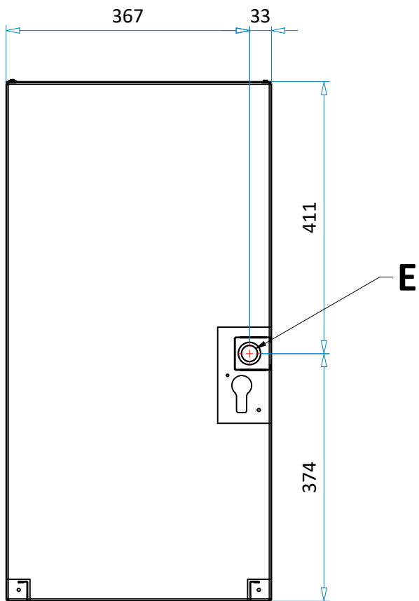
SEZIONE A - A
