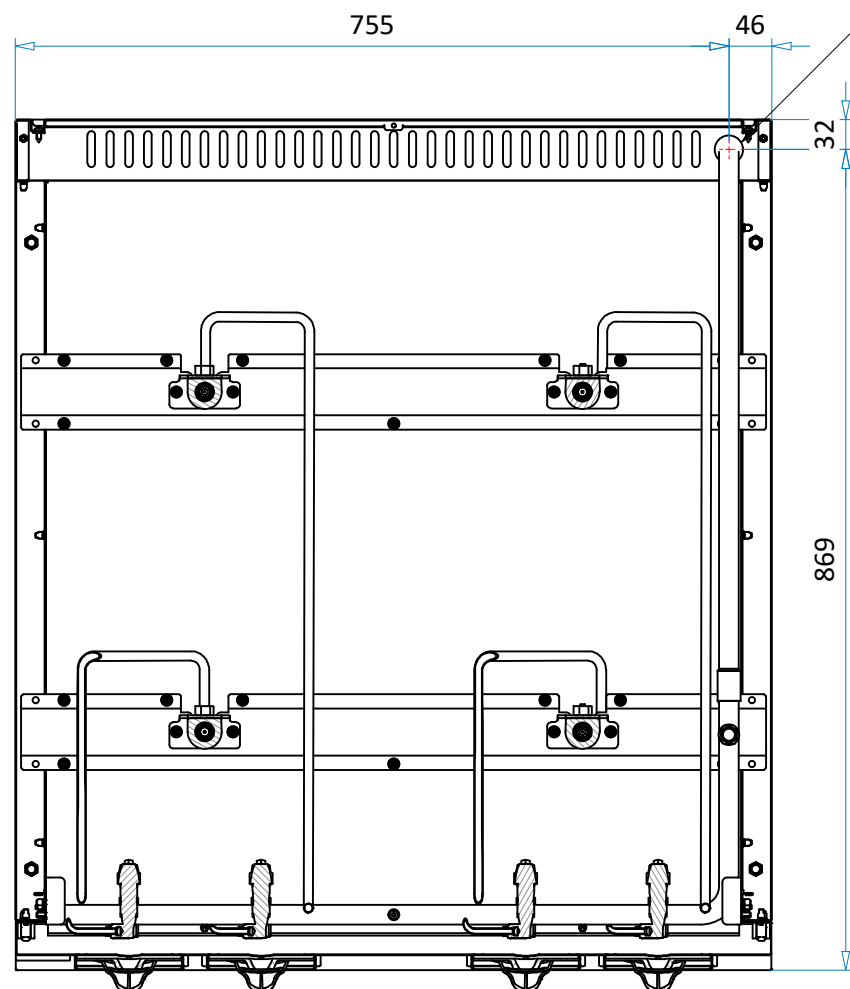
SEZIONE A - A
