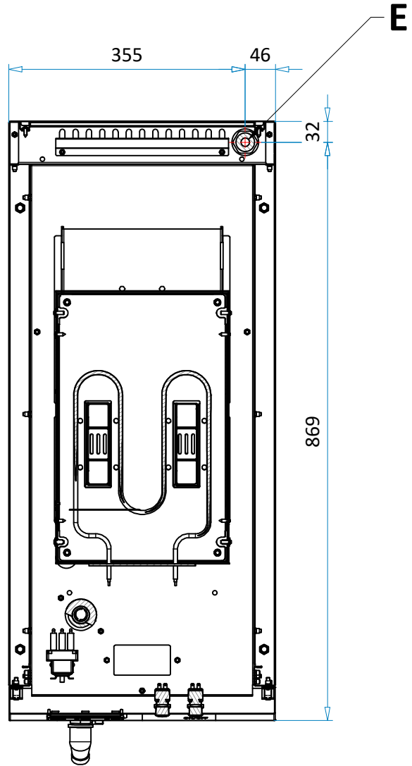
SEZIONE A - A
