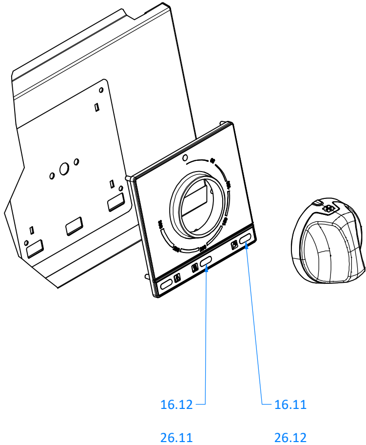
PARTICOLARE B
