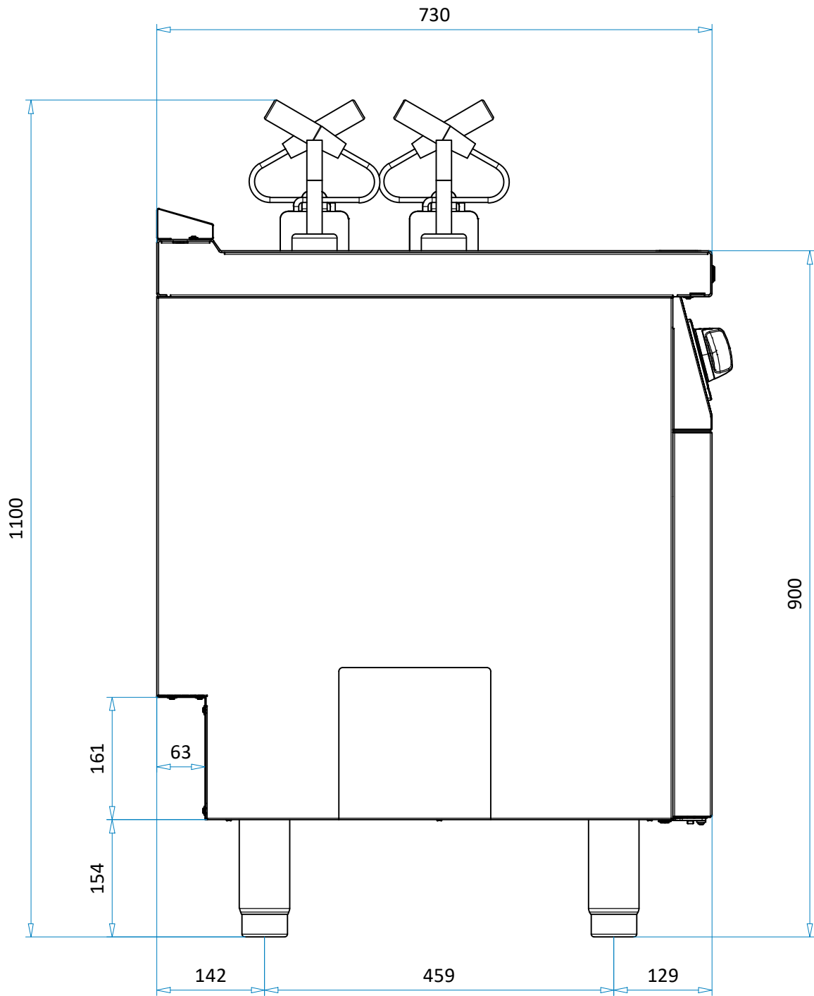
SEZIONE A - A
