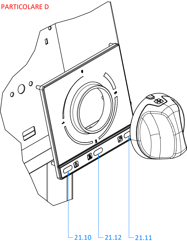
PARTICOLARE D
